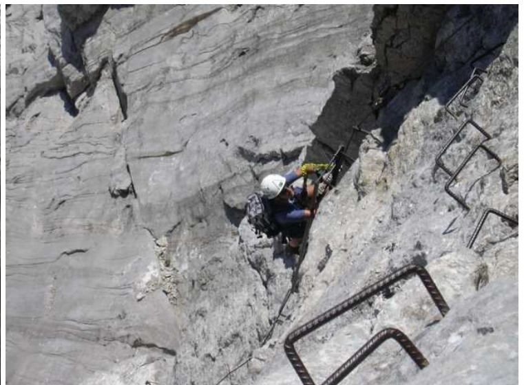
im 2. Steilaufschwung
